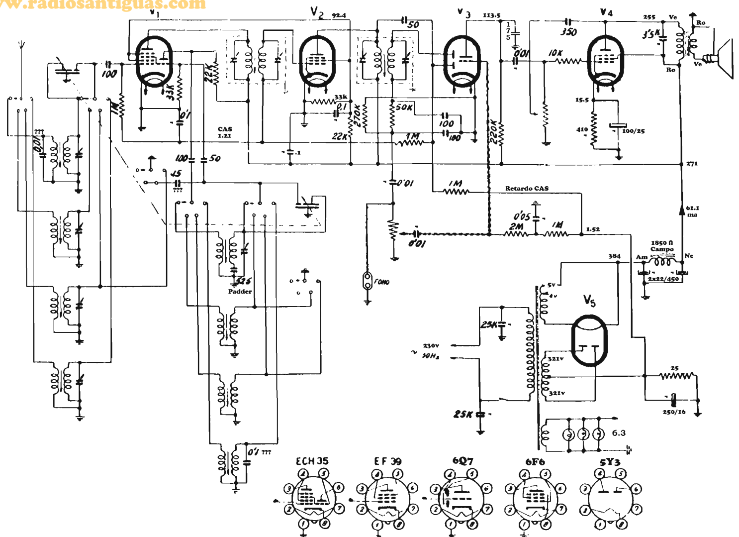
F.I. 470KHz Año 1951 Invicta Saigon 5402 (Modificado)
