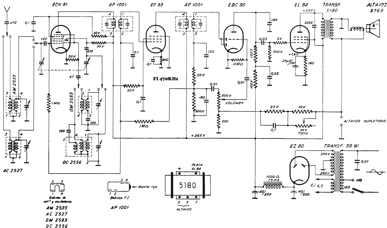
Fig. 1—Esquema del receptor de C. A., con dos válvulas «Miniatura» y tres «Noval».
