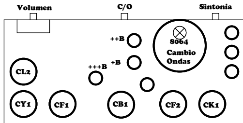
Vista inferior
